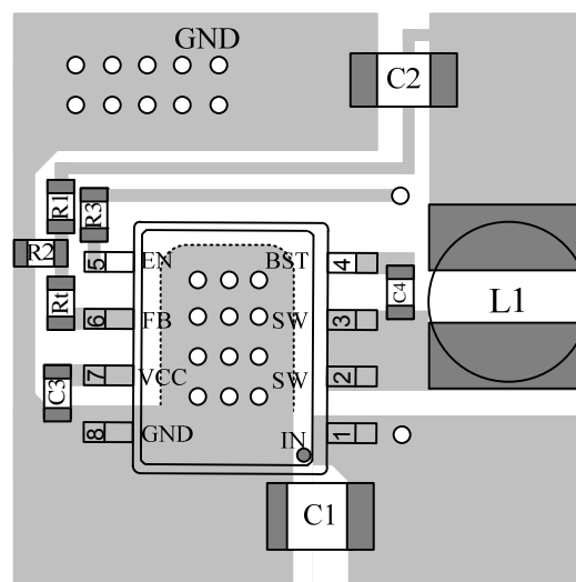
Top Layer
